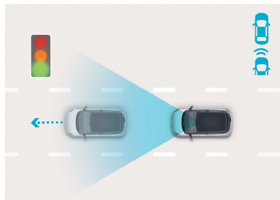
התרעה על התחלת הנסיעה של הרכב מלפנים (LVDA) בזמן עצירה ובמידה ויש רכב מלפנים המערכת תתריע על התחלת הנסיעה של הרכב מלפנים.
